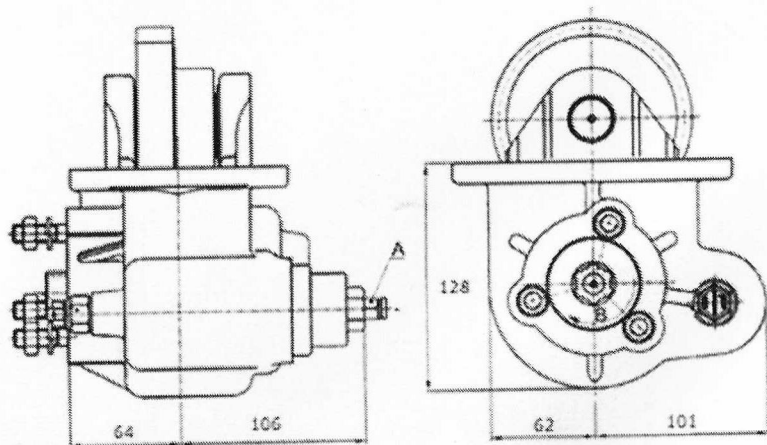
Рис.1 Габаритные и присоединительные размеры HDX M03P1 UNI
