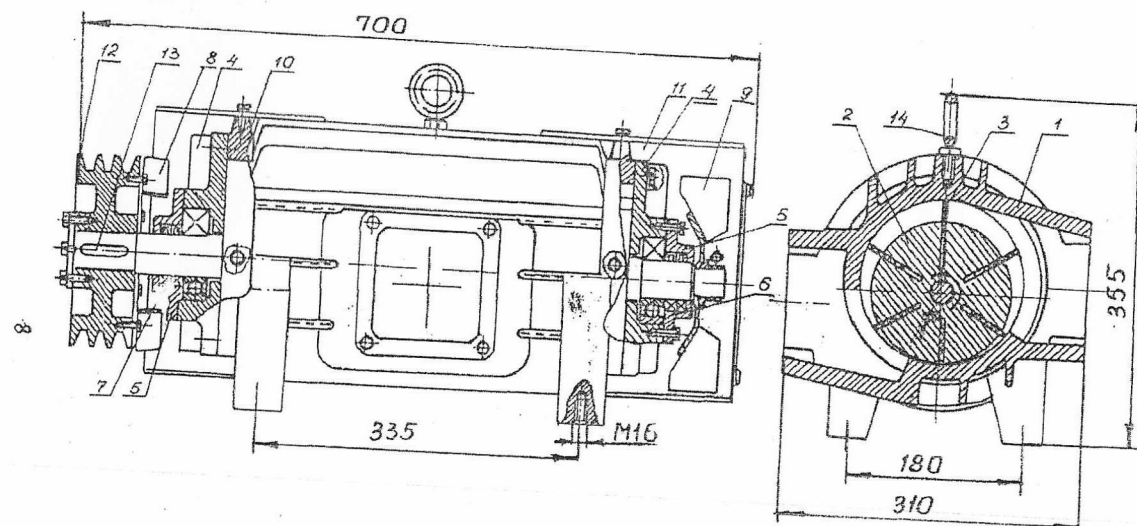
Рисунок 1 – Вакуум-насос.
